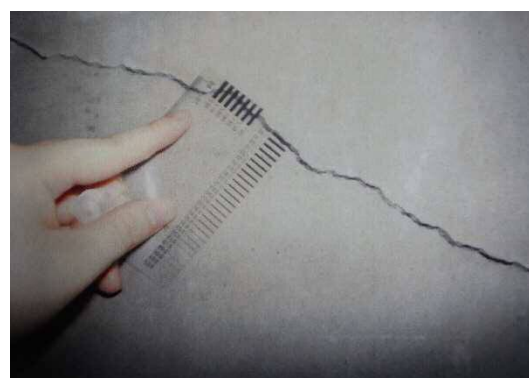
壁のクラック測定
