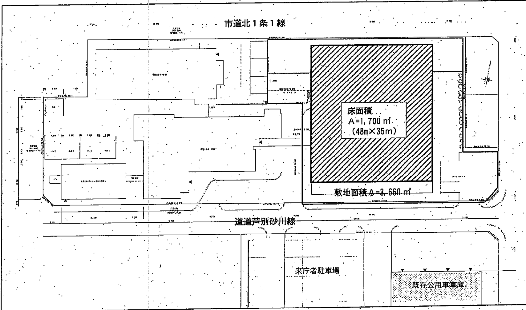
新庁舎建設の床面積を1,700㎡とした場合の敷地配置図
