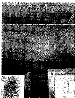
内装梁のひび割れ
